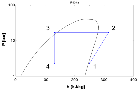
Figura 2 - Diagramma Pressione-Entalpia
