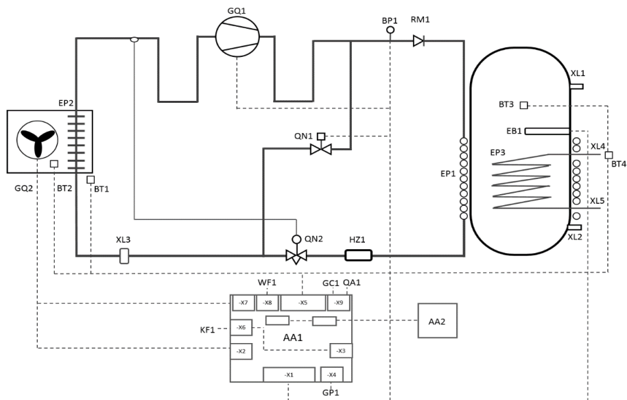
Figura 3 - Diagramma di Processo e Strumentazione
