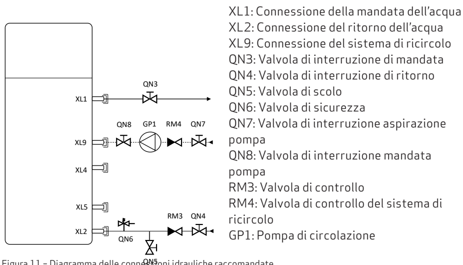
Figura 11 - Diagramma delle connessioni idrauliche raccomandate
