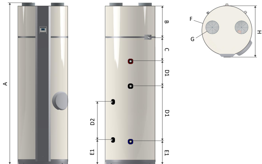
Figura 6 - Dimensioni
