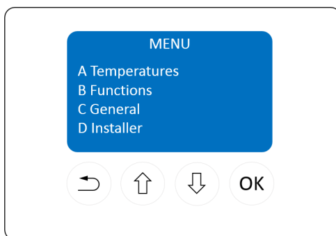
Figura 19 - Menù principale
